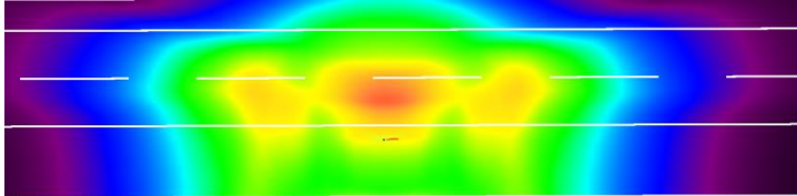
LEVO3 O6R | 53W
