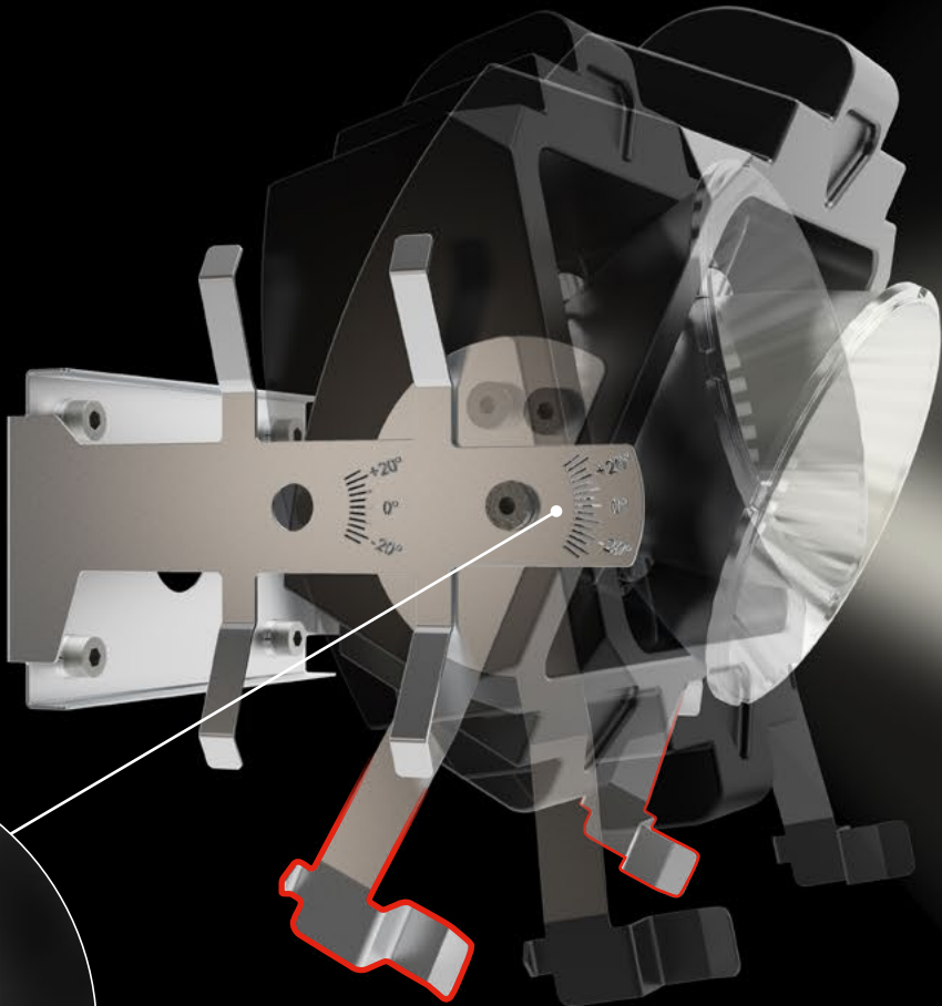
Klammer drücken, Neigungswinkel einstellen und durch loslassen der Klammer den Spot arretieren. So einfach ist die Einstellung der Spots in der neuen CITY ELEMENTS 200.
