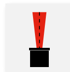
Réflecteur 0% scat Y_{10\%} = 2 \times 6,6^\circ Y_{50\%} = 2 \times 3,6^\circ
